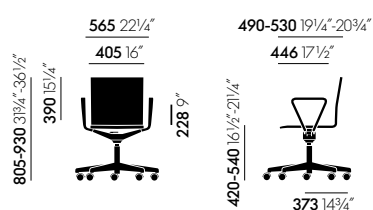
.04, Ateliertstuhl, mit Armlehnen
