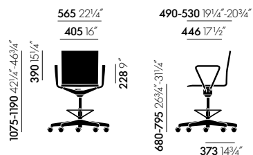
.04 Counter, Counterstuhl, mit Armlehnen
