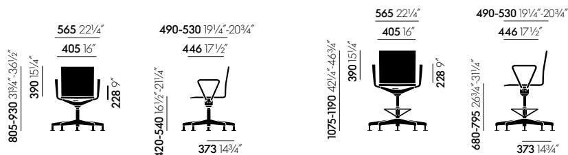
.04, Ateliestuhl, mit Armlehnen
